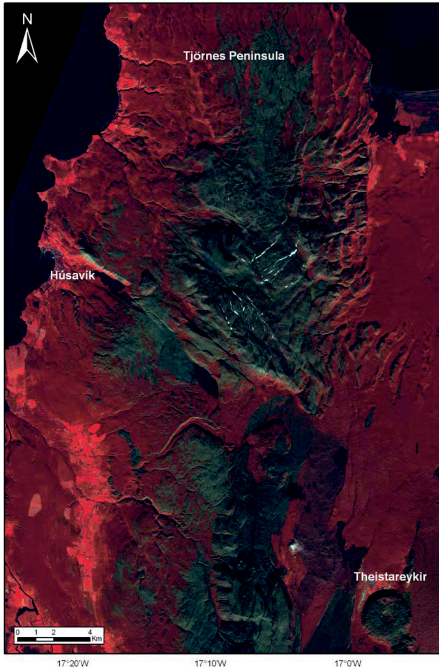
Figure 9. ©SPOT-image of the triple junction formed where the Húsavík-Flatøy Zone merges with the Þeistareykir fissure swarm. – SPOT-gervitunglamynd af þrípunktinum þar sem Húsavíkur-Flatøyjar-sprungubeltið mætir sprungusveim Þeistareykja.
