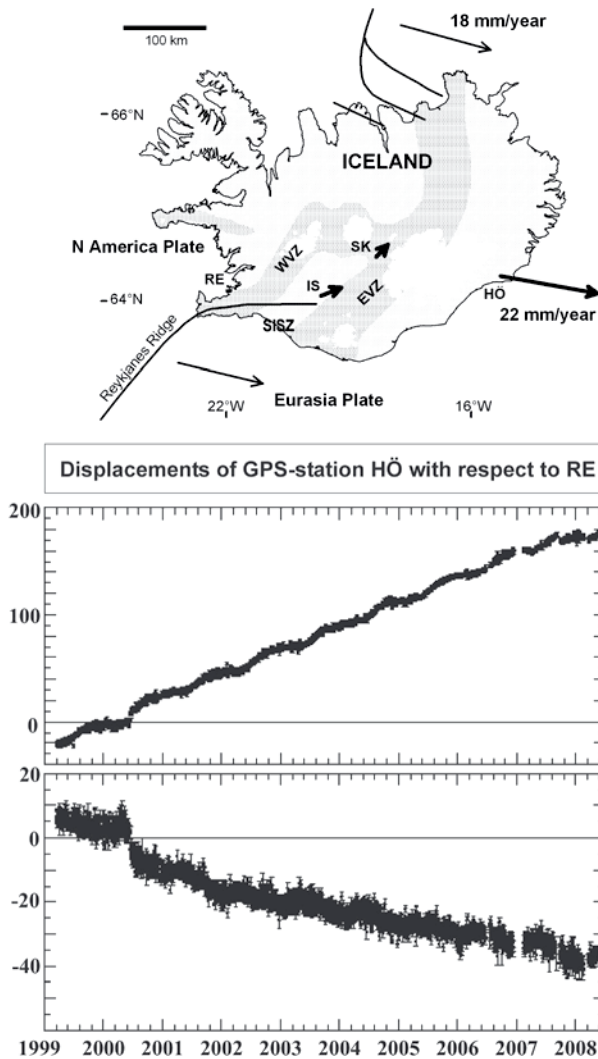
Figure 3. Velocities of the continuous GPS-stations Höfn (HÖ), Skrokkalda (SK), and Ísakoti (IS) with respect to Reykjavík (RE) shown as fat arrows. Thin arrows show the calculated velocity of the Eurasia Plate with respect to the North-America Plate according to the Nuvel 1 model. Time-series of the displacements of the station of Höfn with respect to Reykjavík is shown (data from Halldór Geirsson, Icelandic Meteorological Office). Index map shows the plate boundaries. The velocities of the stations SK and IS are 3 mm/a in direction 50^\circ and 5 mm/a in direction 70^\circ , respectively. – Rekhræði á samfelldu GPS-mælistöðvunum á Höfn í Hornafirði (HÖ), Skrokköldu (SK) og Ísakoti (IS) reiknaður miðað við Reykjavík. Þunnu örvarnar sýna rekhræðann á Evrasíuflekanum miðað við Norður-Ameríkuflekann reiknaðan eftir Nuvel-1-líkaninu fyrir flekarek á jörðinni. Einnig er sýnd færsla sem fall af tíma fyrir stöðina á Höfn í Hornafirði, reiknuð miðað við stöðina í Reykjavík. Kortið sýnir flekaskil-in á Íslandi. Hraði stöðvanna tveggja sem eru á Hreppaflekanum er: Skrokkalda 3 mm/ári í stefnu 50^\circ og Ísakoti 5 mm/ári í stefnu 70^\circ .
